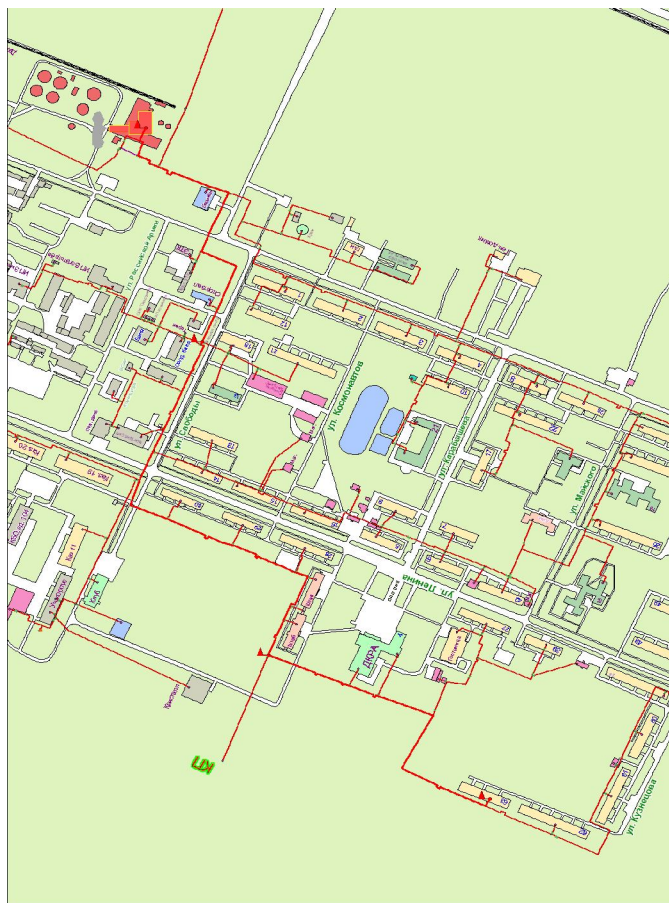
Приложение 1 Путь пьезометрического графика № 2
